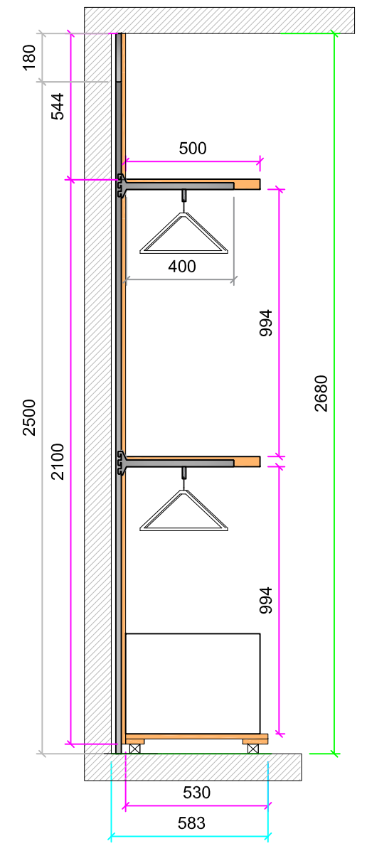
SECCIÓN D-D'
