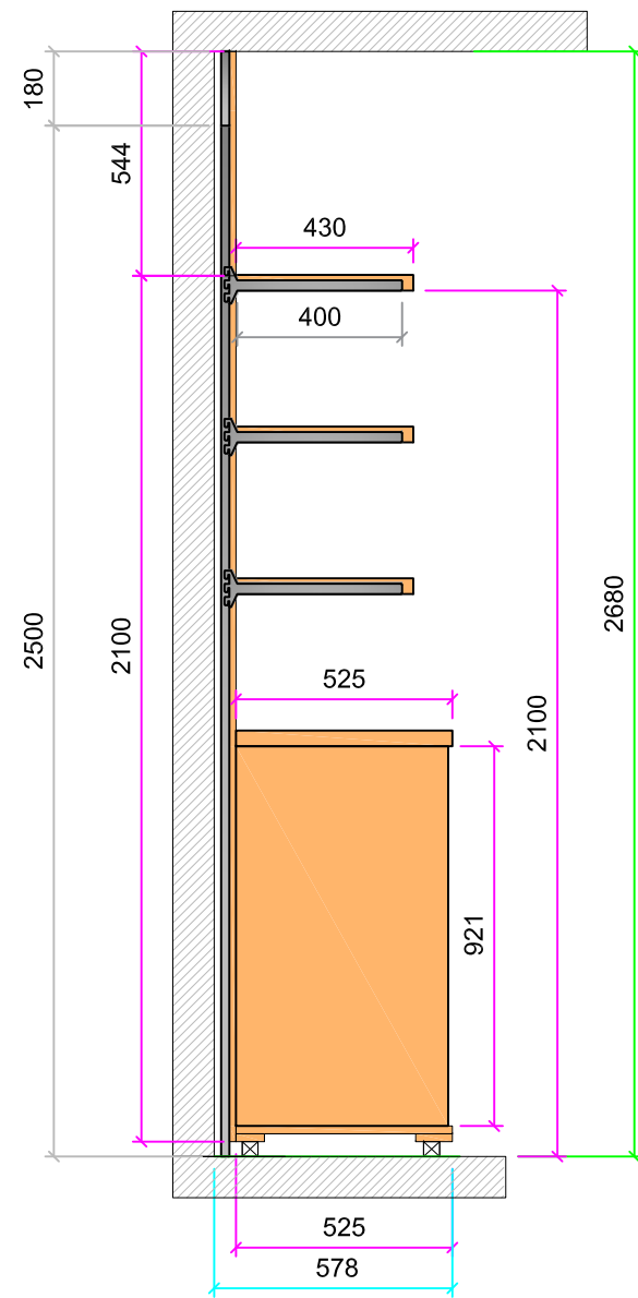
SECCIÓN B-B'
