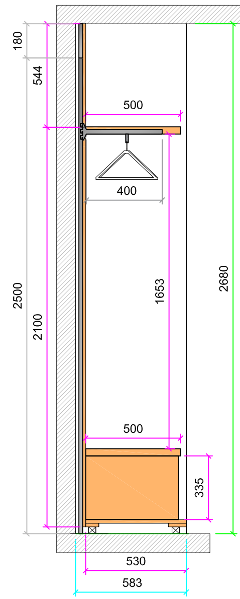
SECCIÓN C-C'
