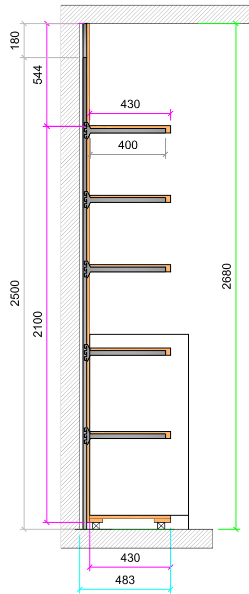
SECCIÓN A-A'
