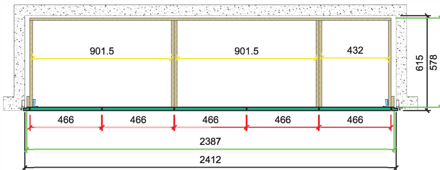
SECCION HORIZONTAL
