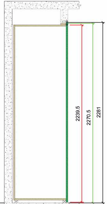
SECCION VERTICAL
